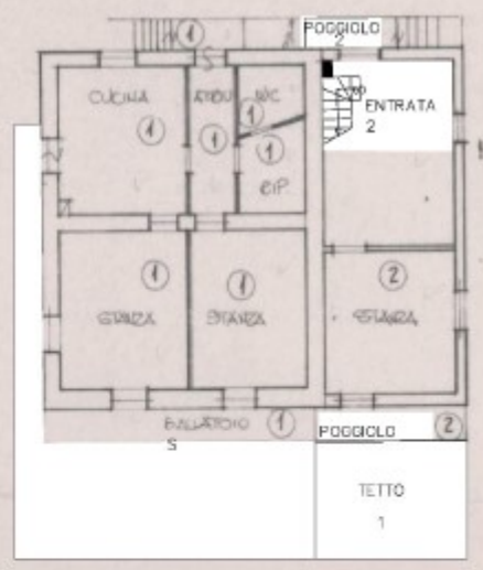
PIANTA PIANO RALZATO
