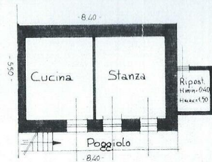
PRIMO PIANO H = 2.60
