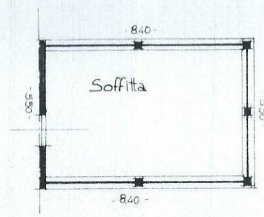
SECONDO PIANO (Soffitta) Hmin = 0.75 Hmax = 2.00
