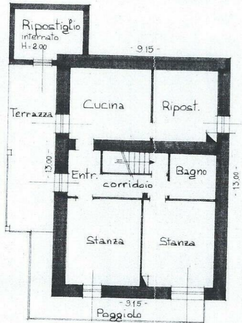
PRIMO PIANO H= 2.50
