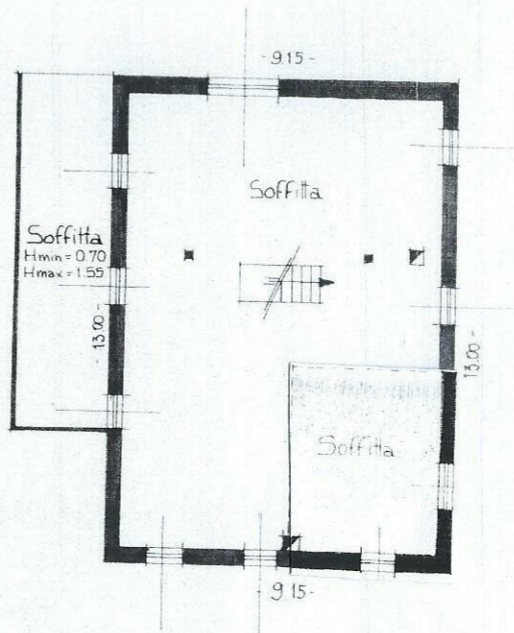
SECONDO PIANO (Sottotetto) Hmin = 1.45 Hmax = 3.35
