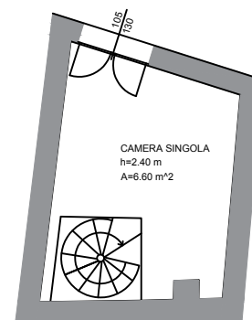
PIANTA CAMERA PIANO SUPERIORE Scala 1:50
