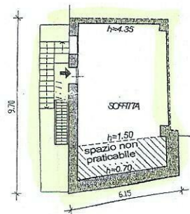
PIANO TERZO - (3) (sottotetto)
